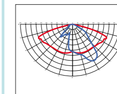
AS7 = Advance street AS7 = Assimétrica de Estrada
