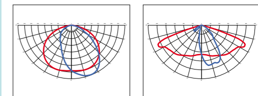
AS7SA = Advance diffuser AS7SA = Assimétrica de Estrada AS8 = Cycling/Narrow street AS8 = Ciclismo/Rua estreita
