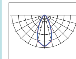
50 = Medium flood 50° 50 = Médio 50°
