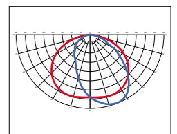
AS7SA = Advance diffuser AS7SA = Assimétrica de Estrada
