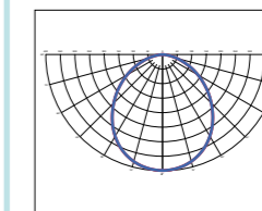
SA = Satin diffuser Difusor SA = Satinado
