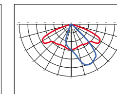
AS9 = Narrow interpost AS9 = Pequenas inter distâncias
