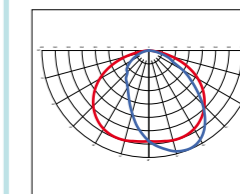
AS7SA = Advance diffuser AS7SA = Assimétrica de Estrada
